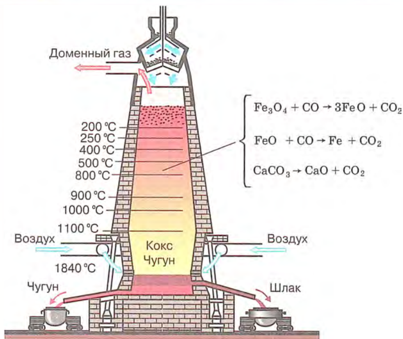
Рис. 46. Доменная печь
