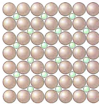
Рис. 25. Структура слоя атомарного азота на поверхности грани железа
