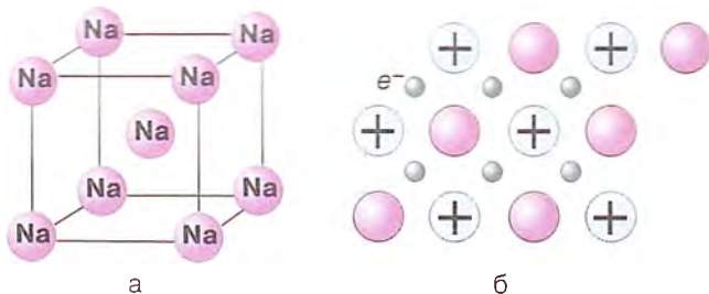
Рис. 15. Элементарная ячейка натрия (а); сдвиг слоёв в металлическом кристалле не приводит к его разрушению (б)
