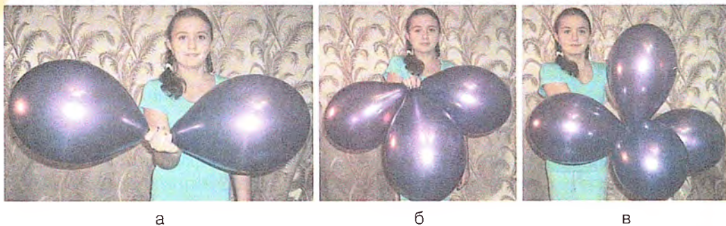
Рис. 12. Скреплённые воздушные шарики ориентируются в пространстве подобно электронным орбиталям: а — два шарика (линейное расположение); б — три шарика (плоский треугольник); в — четыре шарика (тетраэдр)
