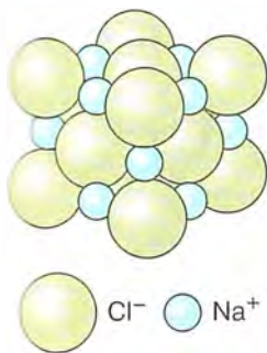
Рис. 16. Ионный кристалл хлорида натрия (слева); разрушение ионного кристалла при сдвигании слоёв ионов (справа)
