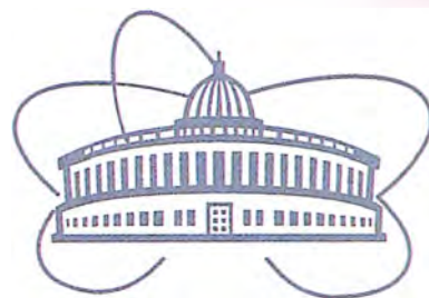
Рис. 6. Эмблема Объединённого института ядерных исследований
