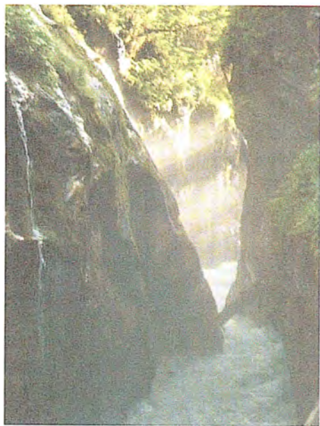
Рис. 27. Эффект Тиндаля (рассеивание света при прохождении его через туман)
