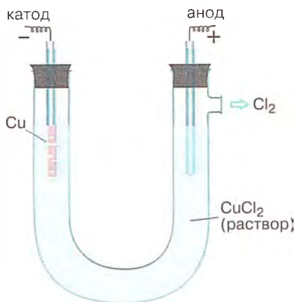
Рис. 36. Электролиз раствора хлорида меди(II)
