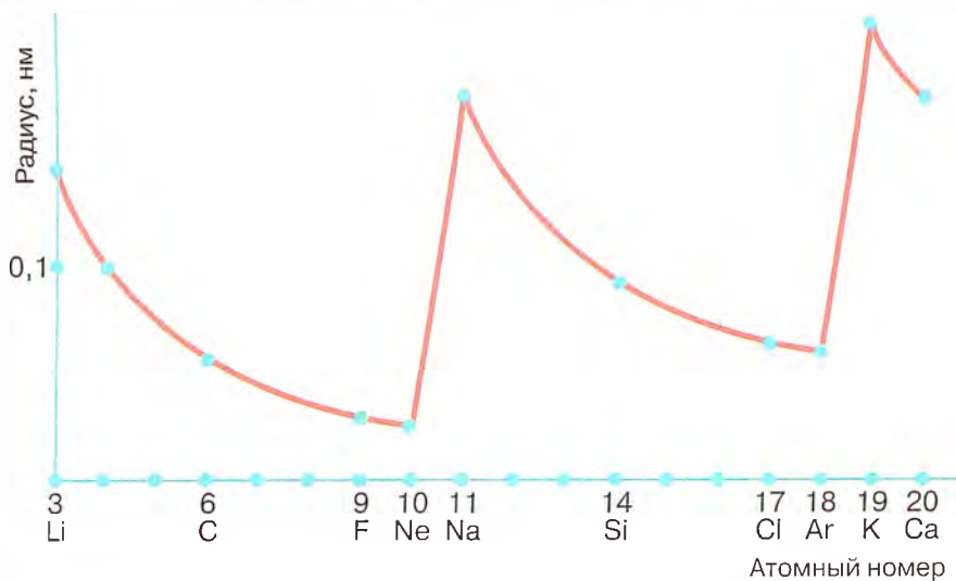
Рис. 8. Изменение атомных радиусов от лития до кальция
