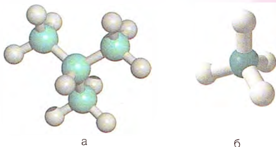
Рис. 22. Шаростержневые модели гомологов — бутана (а) и метана (б)
