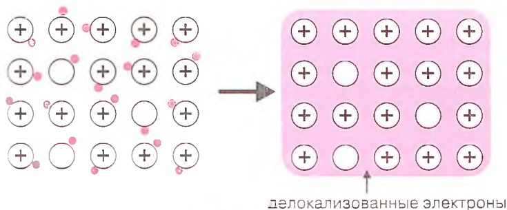
Рис. 10. Образование металлической связи
