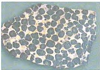
Рис. 42. Хромистый железняк
