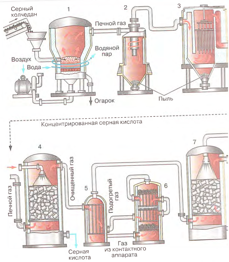
Рис. 45. Производство серной кислоты: 1 — печь для обжига пирита; 2 — циклон; 3 — электрофильтр; 4 — сушильная башня; 5 — теплообменник; 6 — контактный аппарат; 7 — поглотительная башня
